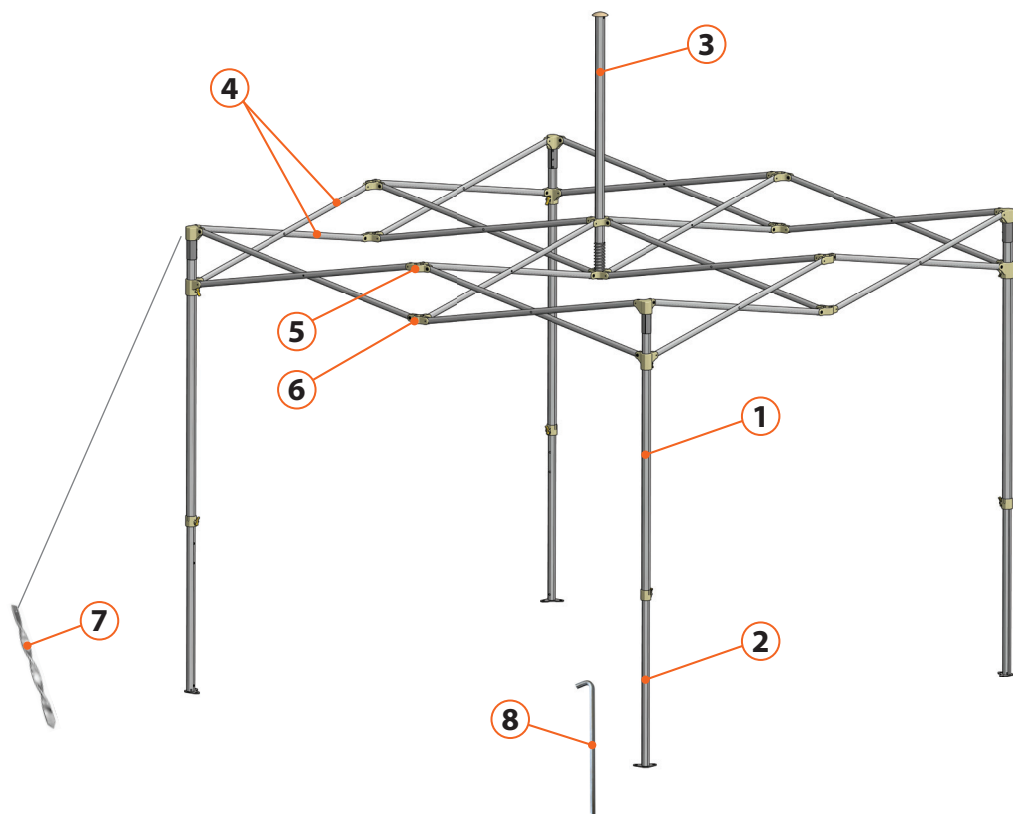
Rys. 1. Wykaz części zamiennych
